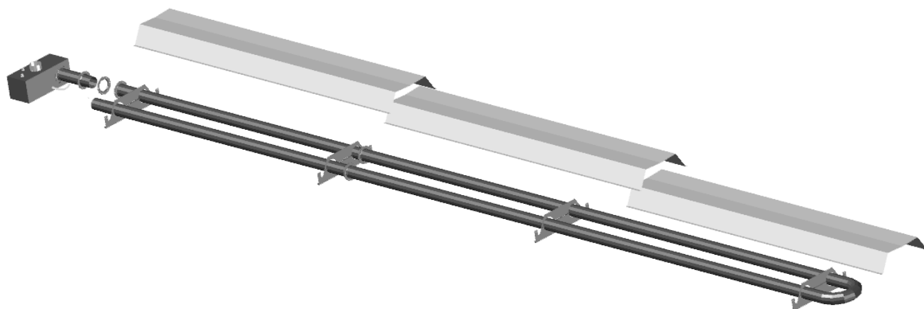
RYS. 18. Montaż ekranów promiennika.
