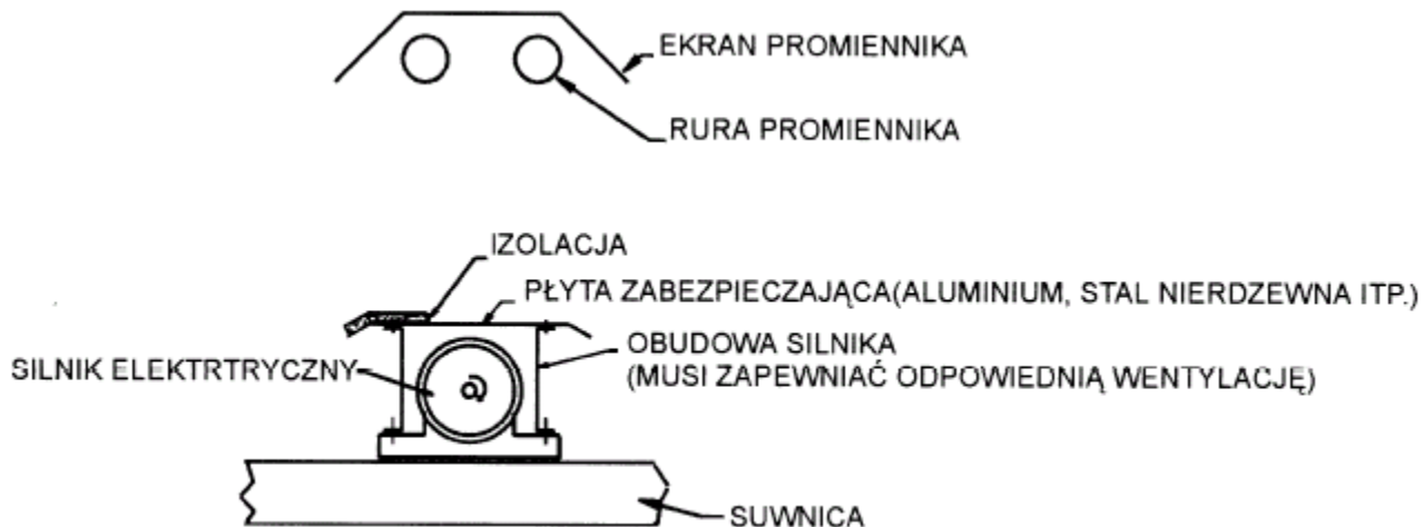
RYS. 15 Przykładowy sposób izolowania silnika suwnicy
